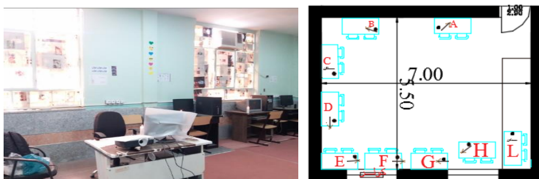
شکل 4- کلاس تحت آزمون: پلان کلاس و نقاط آزمون (راست) و شکل کلاس (چپ) Fig. 4- The studied classroom: plan and the tested points (right) and inner view (left)
