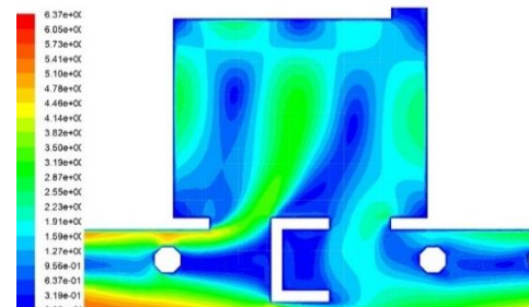
k. کانتورهای سرعت جریان هوای داخل: تیغه وسط چسبیده به پنجره غربی و در باز
