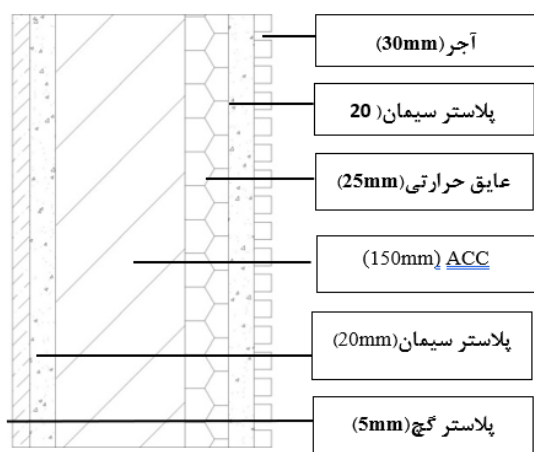
شکل 17- لایه بندی دیوار خارجی Fig.17- External wall layering
