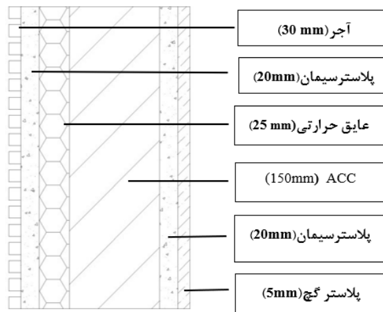
شکل 16- لایه بندی دیوار داخلی Fig.16- Inner wall layering
