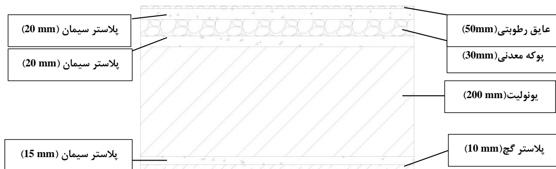
شکل 18- لایه بندی سقف Fig.18- Roof layering
