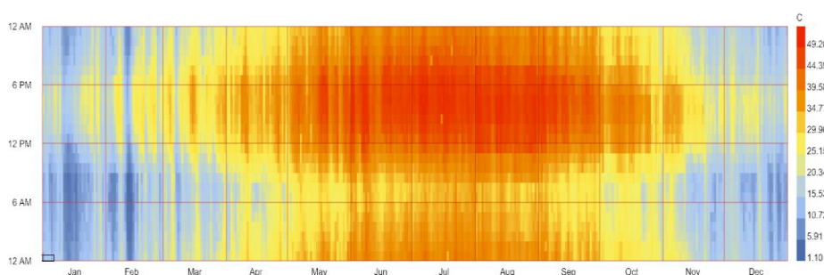
شکل 7-دمای سالانه هوای خشک در شهرستان اهواز
