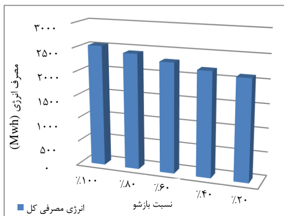
شکل ۸- انرژی مصرفی کل در نسبت‌های بازشوی مختلف در شهر تهران
