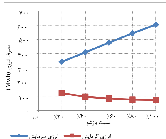
شکل ۱۱- انرژی سرمایشی و گرمایشی در نسبت‌های بازشوی مختلف در شهر تهران
