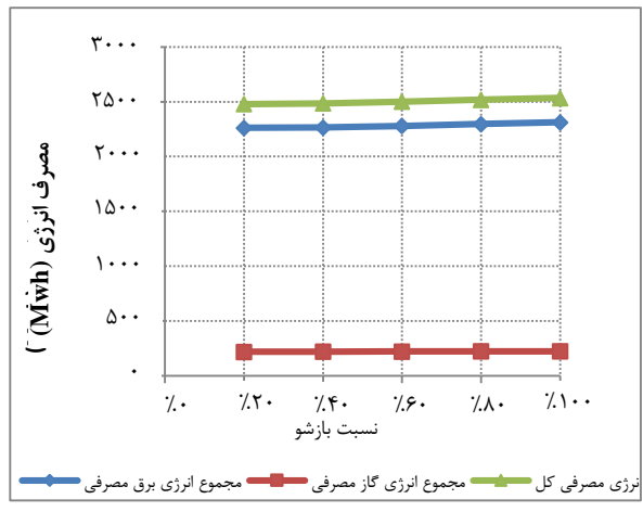
شکل ۶- تغییرات انرژی برق، گاز و انرژی مصرفی کل در نسبت‌های بازشوی مختلف جداره شمالی
