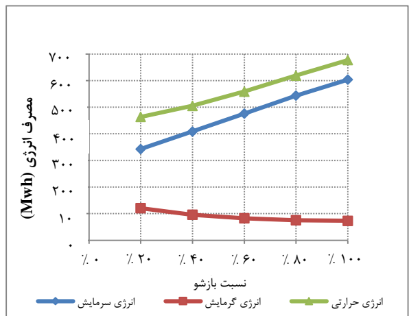
شکل ۴- تغییرات انرژی گرمایش، سرمایش و انرژی حرارتی در نسبت‌های بازشوی مختلف
