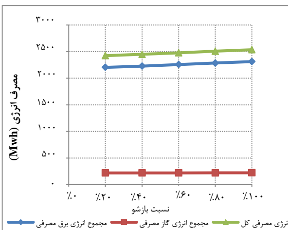
شکل ۵- تغییرات انرژی برق، گاز و انرژی مصرفی کل در نسبت‌های بازشوی مختلف جداره غربی
