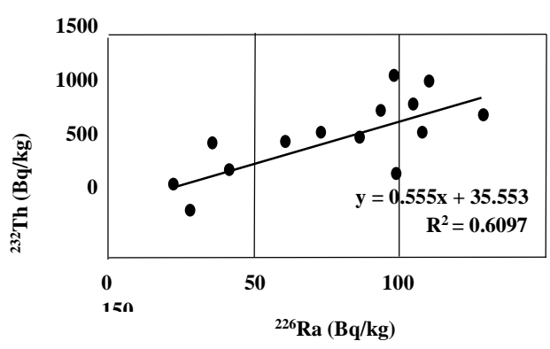
شکل 5- همبستگی مثبت بین میانگین شدت فعالیت تشعشعی ایزوتوپ‌های ^{232}\text{Th} و ^{40}\text{K} (تصویر A)، ایزوتوپ‌های ^{226}\text{Ra} و ^{40}\text{K} (تصویر B) و ایزوتوپ‌های ^{226}\text{Ra} و ^{232}\text{Th} (تصویر C) برای سنگ‌های پلوتونیک (عمدتاً گرانیتوئید) که در 13 منطقه از ایران رخنمون دارند.
